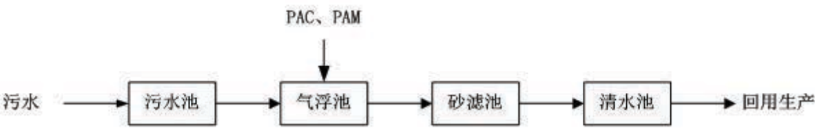
污水处理流程图
